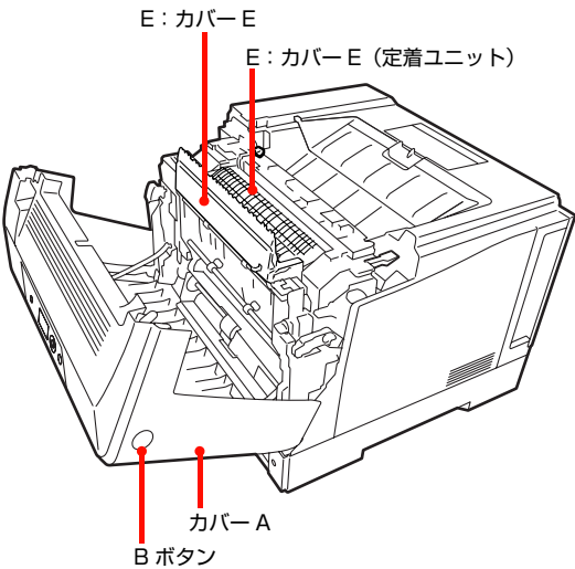
B ボタンを押してカバー A を開いた状態
