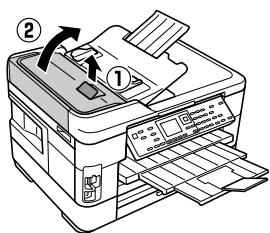
レバーを引きながら ADF カバーを開ける
