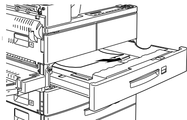
図はカセット 1 の場合 (カセット 2・3 も同様)
