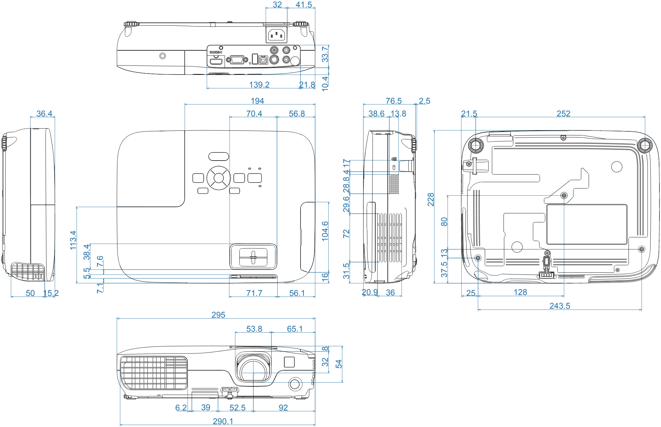
EB-W10/X10/S10本体外観図
