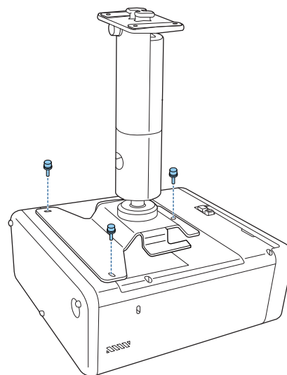
无投影机板
