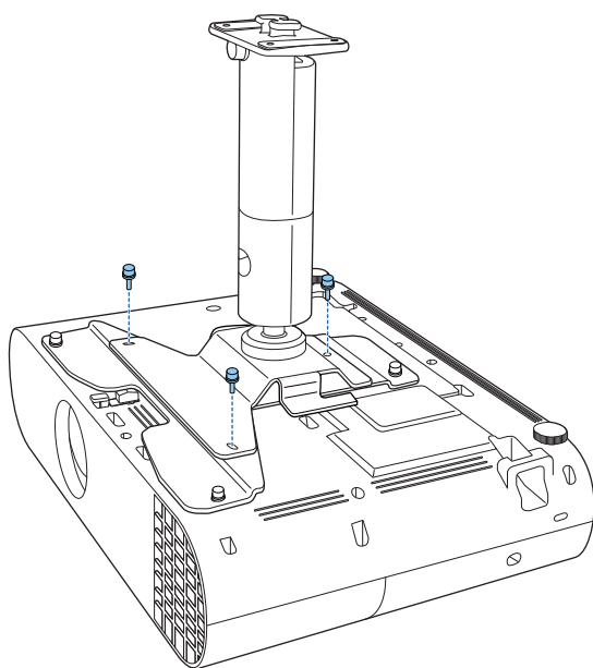
带投影机板
