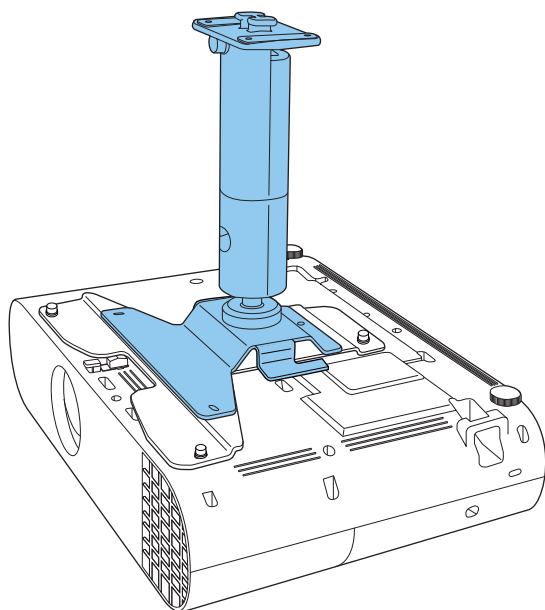
有投影機板
