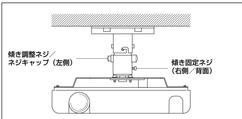
設置正面図
