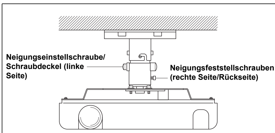
Frontansicht
