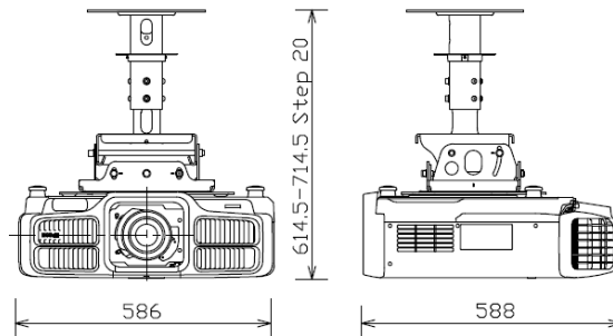
<ELPMB48 装着図>
