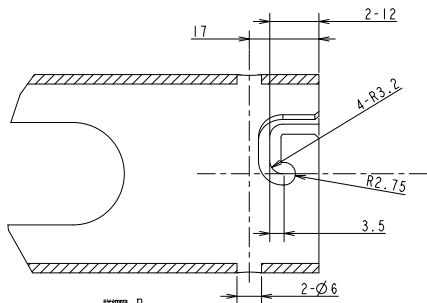
詳細 B スケール 1.000
