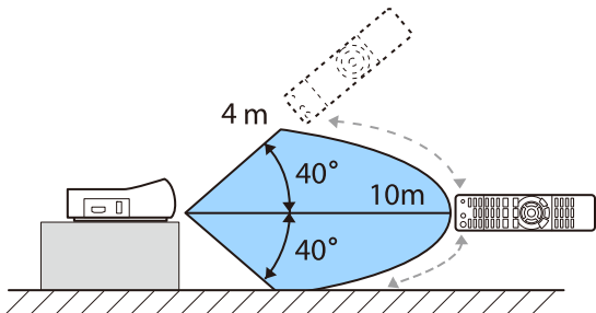
操作可能範囲（上下）
