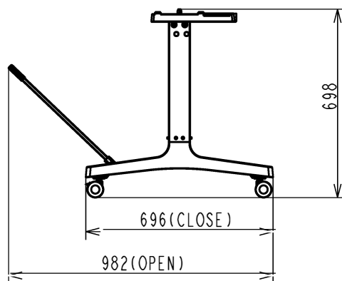
<側面>
