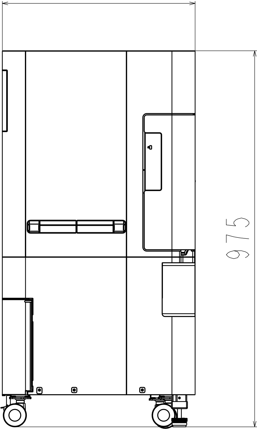
<側面>
