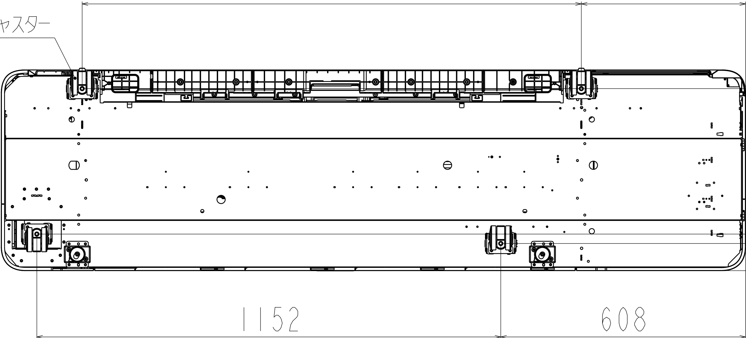
<底面>
