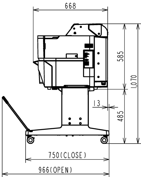
<側面>
