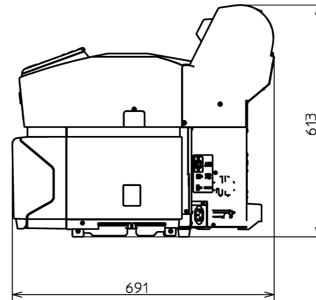
<側面>
