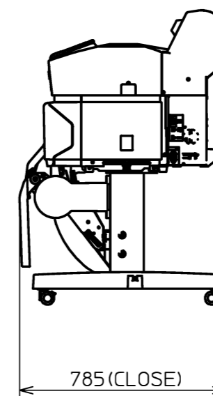
<側面>
