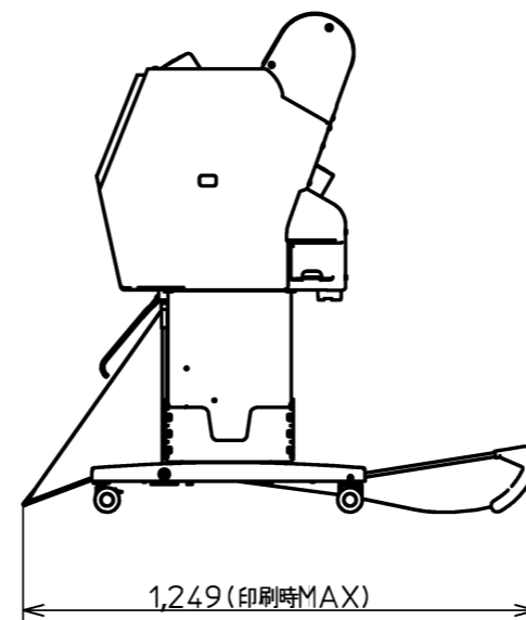
<側面>
