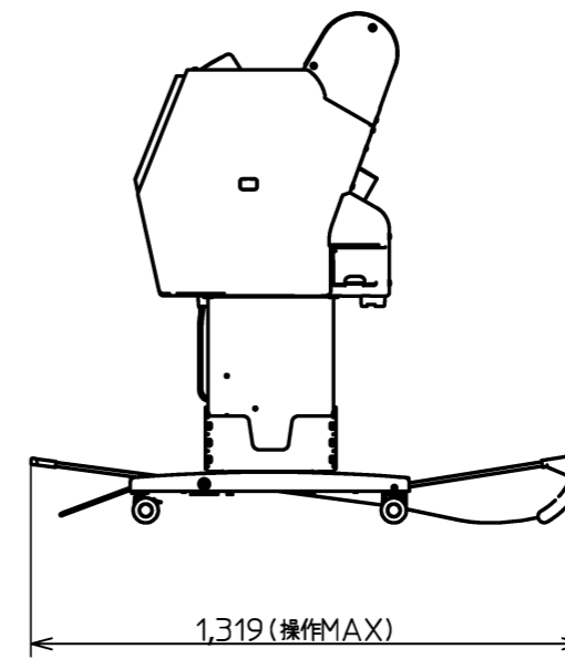
<側面>
