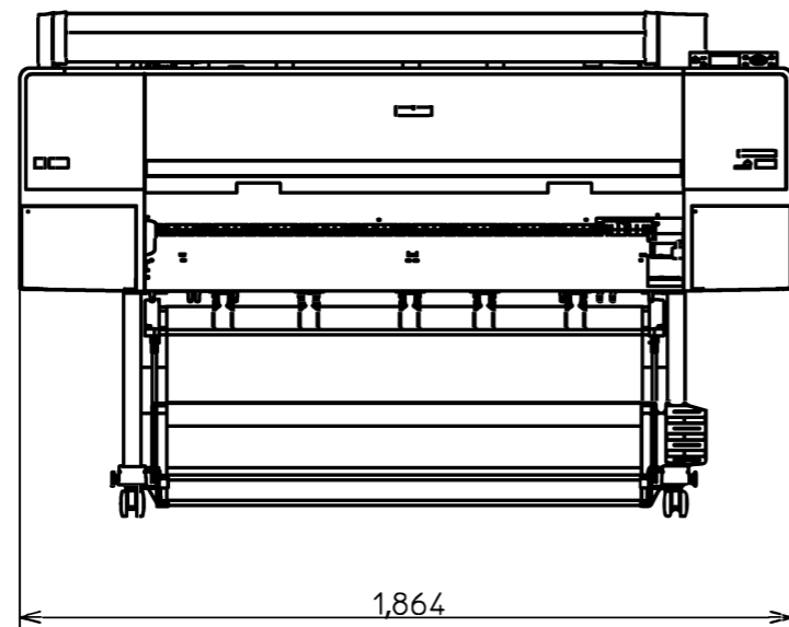
<正面>
