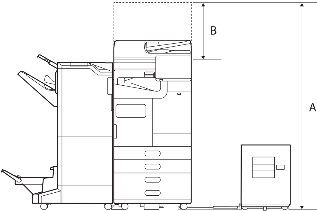
ステープルフィニッシャー装着時 正面
