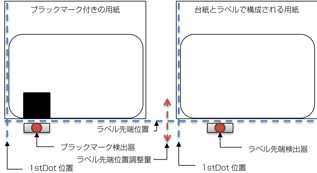
図 2.4.3 ラベル先端位置検出方法
