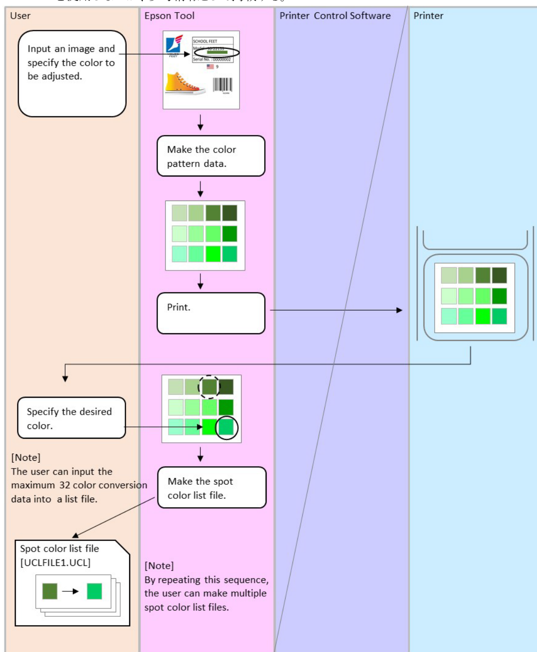
Figure 4.5.6-4 特色リストファイルの作成
