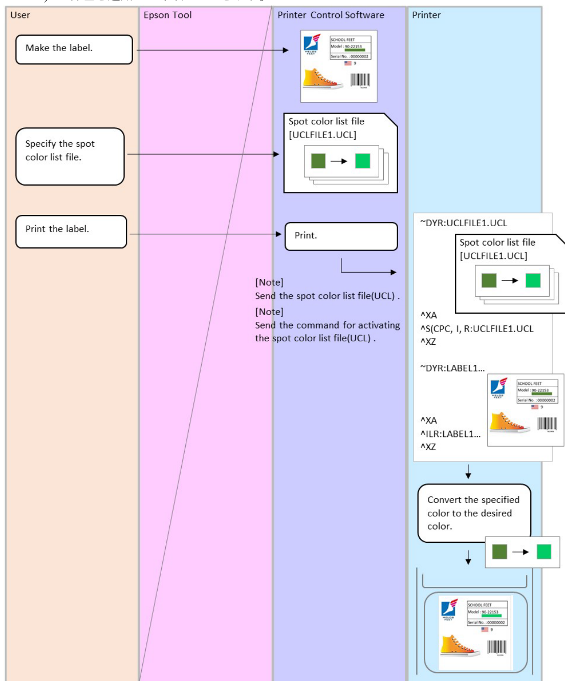
Figure 4.5.6-5 特色を適用した印刷
