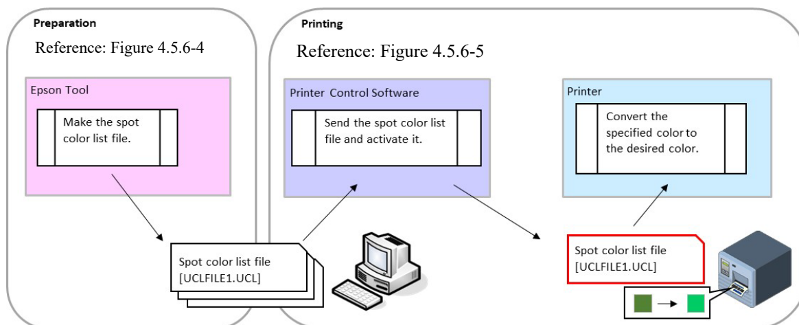
Figure 4.5.6-2 特色調整概フロー
