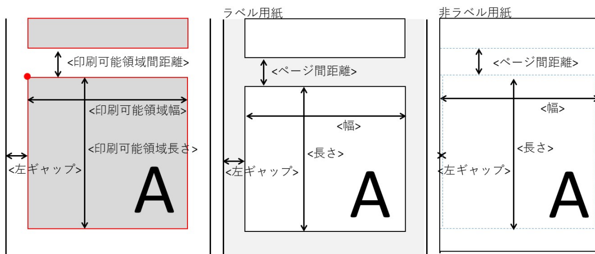
Figure 4.3.2-1 印刷可能領域、ユーザー入力項目と用紙仕様
