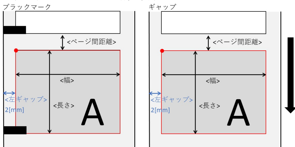
Figure 4.3.2-2 ダイカットラベルレイアウト
