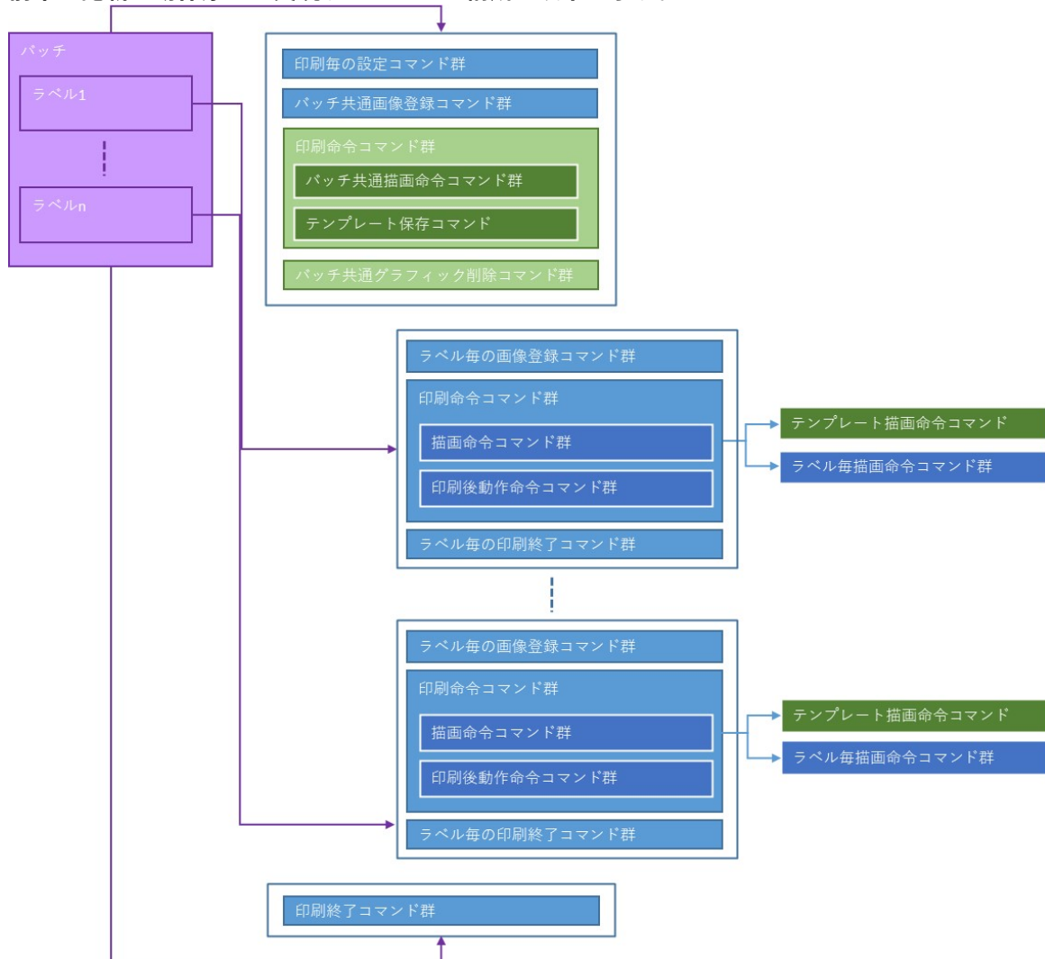
Figure5.2.2-1 コマンド構成
