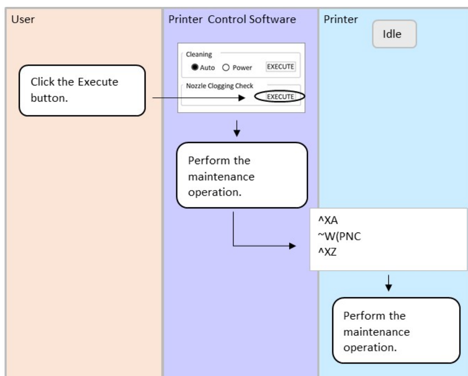
Figure 8-1 プリンターメンテナンスシーケンス
