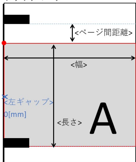
Figure 4.3.2-4 連続紙レイアウト
