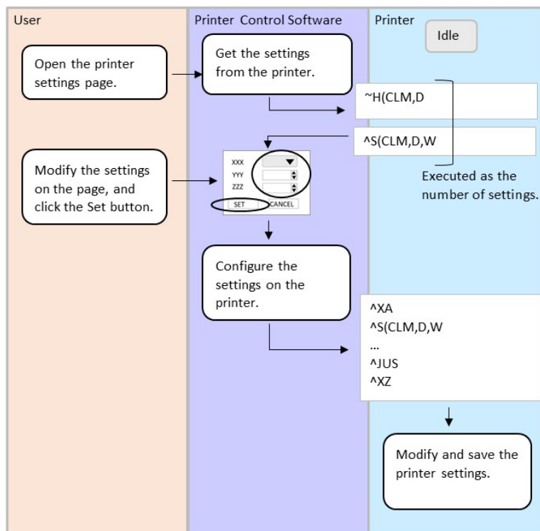
Figure 6-1 プリンター設定シーケンス
