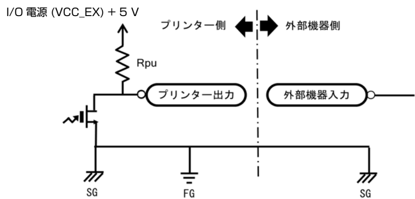
入出力信号(I/O 電源 (VCC_EX)/SG 分離時)の仕様
