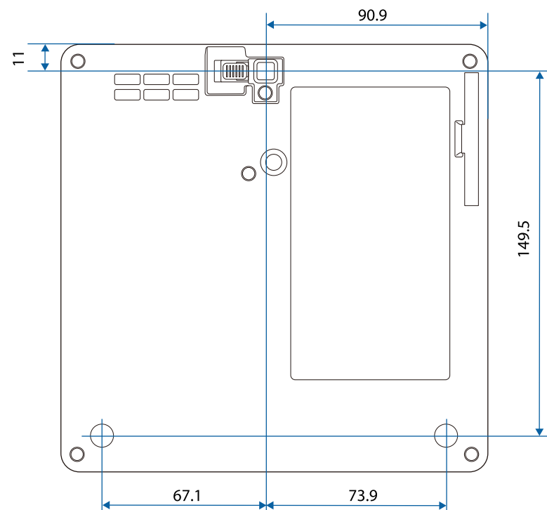
② レンズ中心から天吊り固定部までの寸法
