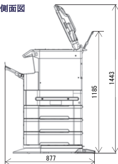
側面図
